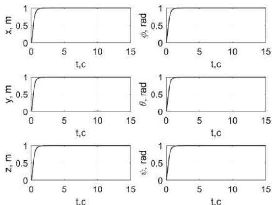
Рис. 2. Переходные процессы системы при номинальных значениях аэродинамических коэффициентов
