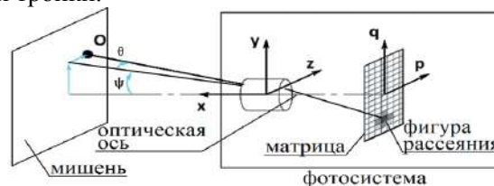
Рис.1. Системы координат, применяемые для расчёта калибровочных характеристик.
