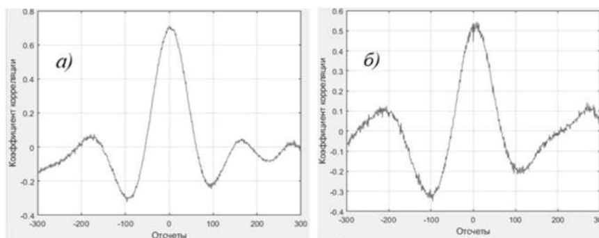
Рис. 3. Корреляция сигналов до (слева) и после (справа) учета коэффициентов перераспределения энергии
