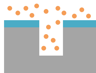
Рис. 1. Схематическое изображение Bosch процесса
