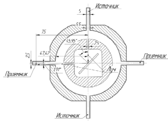
Рис. 2. Схема расположения измерительных элементов
