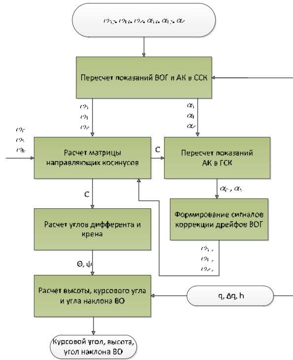
Рисунок 2 – Блок-схема алгоритма
