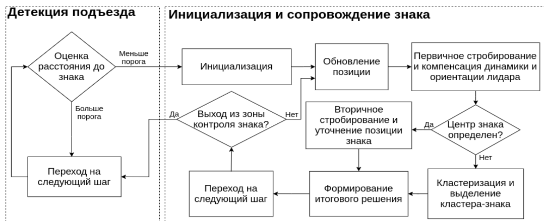
Рис. 1. Блок-схема алгоритма
