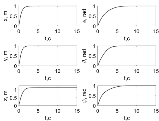
Рис. 3. Переходные процессы системы при увеличении до 3 раз значений аэродинамических коэффициентов
