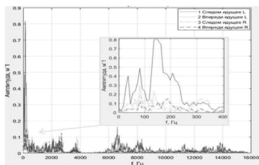
Рис. 2. Амплитудно-частотный спектр сигнала
