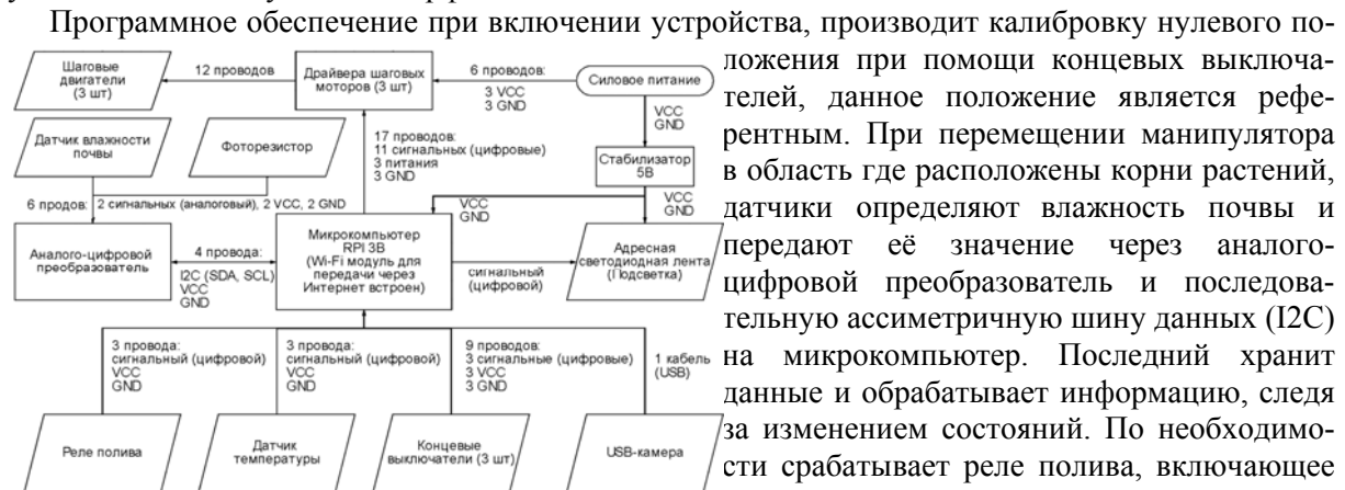
Рис. 3. Схема интерфейсов подключения устройств к микрокомпьютеру
