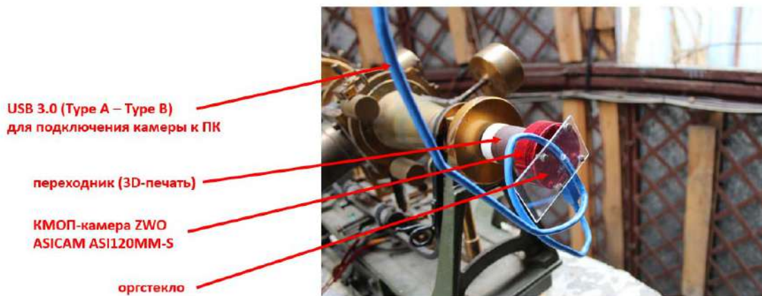
Рис. 2. Модернизированный пассажирный инструмент Vamberg
