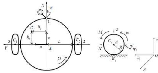
Рис. 1 Кинематическая схема робота
