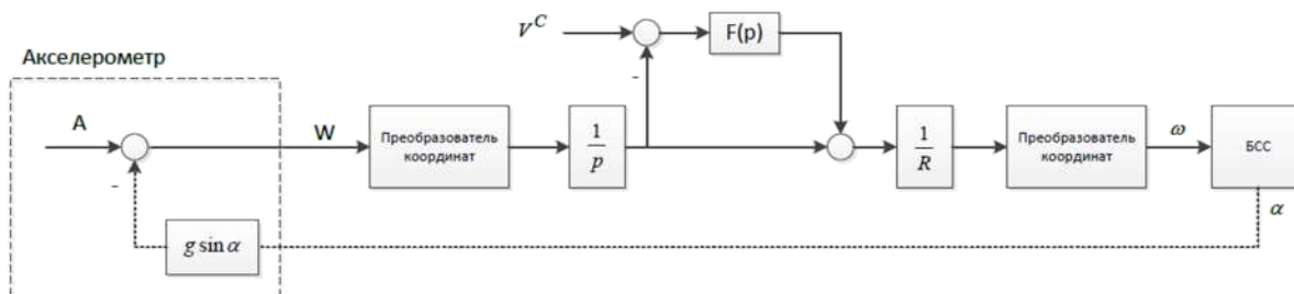
Рис. 1. Структурная схема системы управления гиросtabilизатором, где V^C – составляющая линейной скорости в горизонтальной системе координат, определяемая по показаниям внешнего источника, F(p) – демпфирующий фильтр шулеровских колебаний, R – радиус Земли, \omega – угловая скорость погрешности стабилизации в приборной системе координат.
