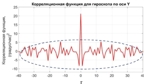
Рис. 1. Корреляционная функция сигнала гироскопа
